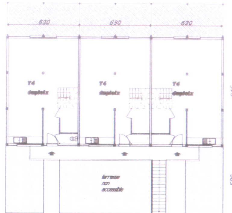
PLAN ETAGE
