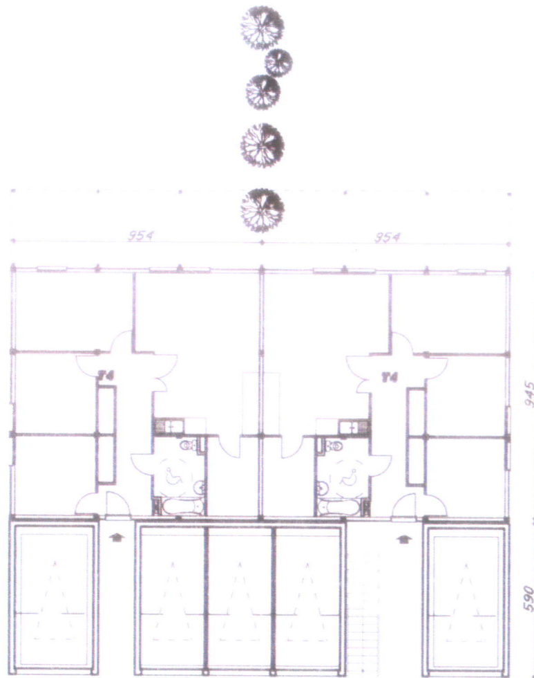
PLAN REZ DE JARDIN
