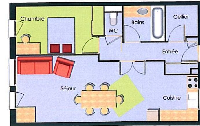
APPARTEMENT T2 (COLLECTIF)
