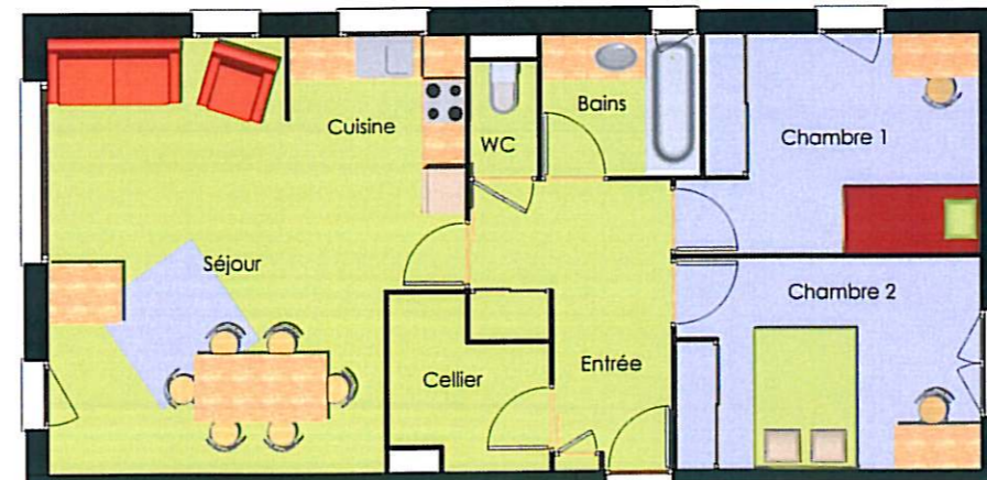
APPARTEMENT T3 (COLLECTIF)
